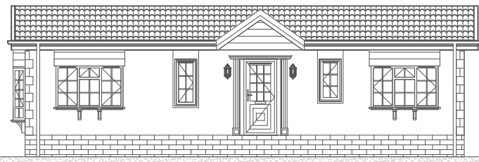
A Elevation
